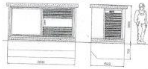
Pohľad na trafostanicu M 1:50
